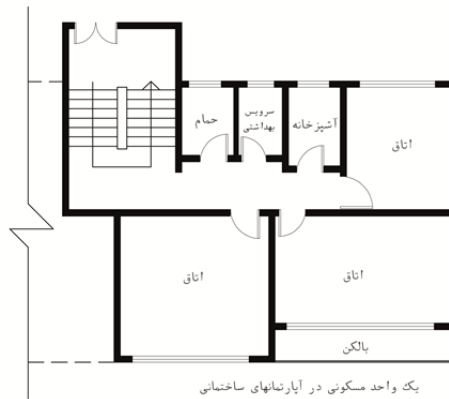
تصویر ۱۴: پلان واحد مسکونی آپارتمان کوی کن (منبع: کیاکجوری، ۱۳۵۱: ۱۴)
