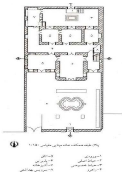
تصویر ۳: پلان همکف خانه مینایی
