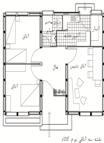
تصویر ۹: نقشه خانه سه اتاقی در نارمک (منبع: خدایار، ۱۳۳۶: ۲۰)
